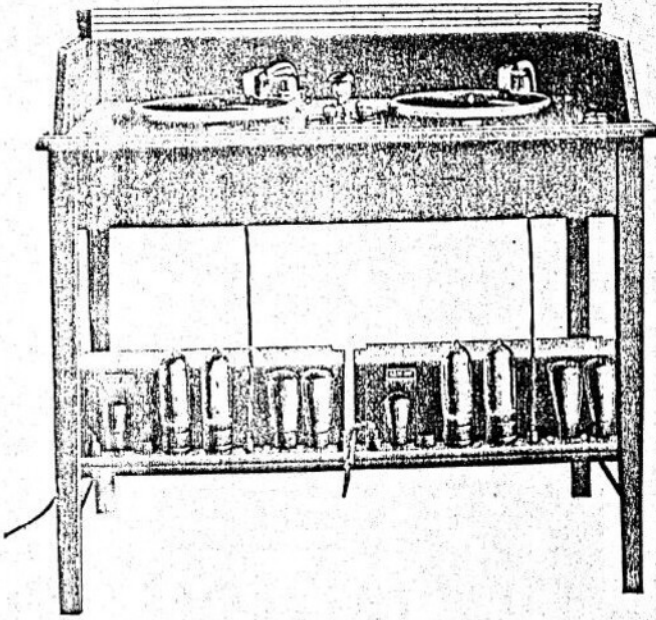
Pantofon No. 511 Sıkleti - 164 kilo netto
